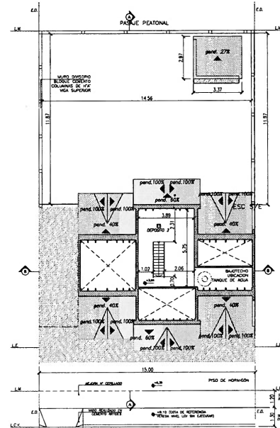
PLANTA ALTA NIVE +1.60 / ESC 1:100
