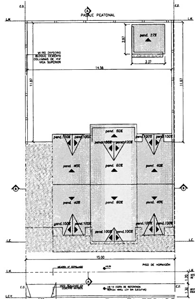
PLANTA TECHOS NIVE +2.10 / ESC 1:100
