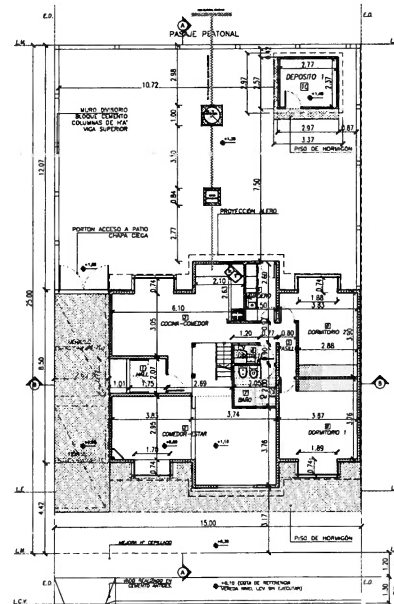
PLANTA BAJA NAVE +0.10 / ESC 1:100
