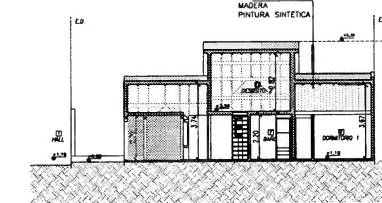
CORTE B-B ESC 1:100
