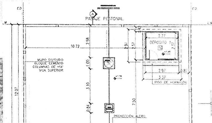
Esquema respecto a ejes.
