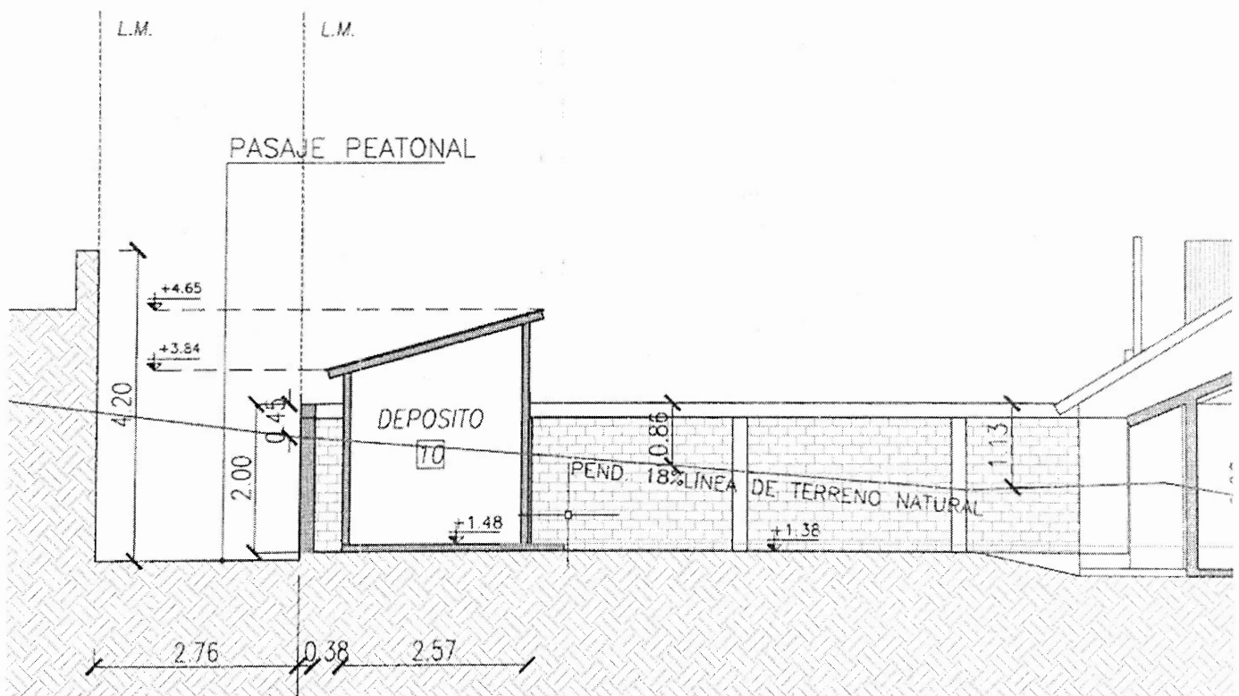
Esquema de situación respecto a terreno posterior y L.T.Nat.
