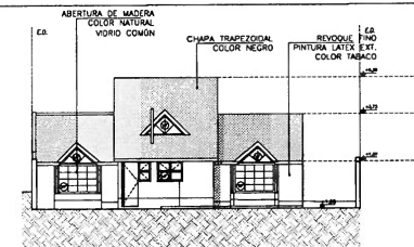
VISTA POSTERIOR ESC 1:100
