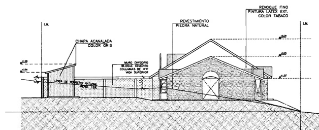
VISTA LATERAL IZQUIERDA ESC 1:100
