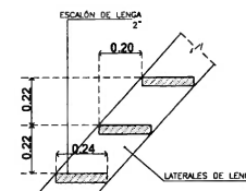
SECCIÓN PARCIAL DETALLE ESCALERA
